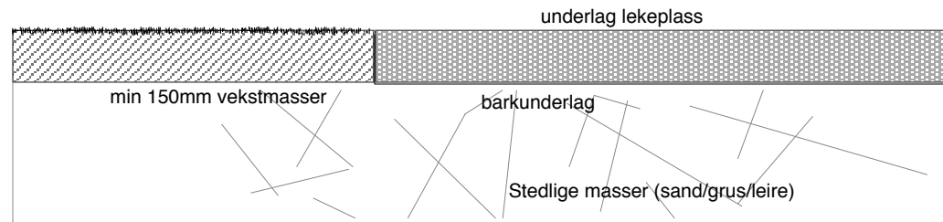
snitt 1 - lekeplass
