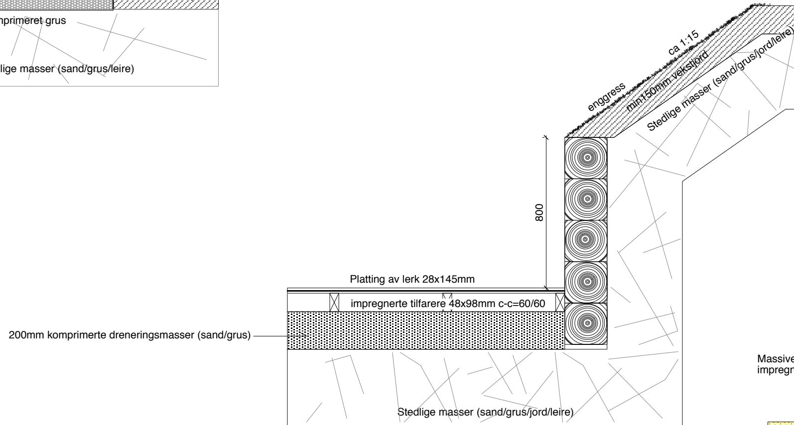
snitt 4 - treplattung
