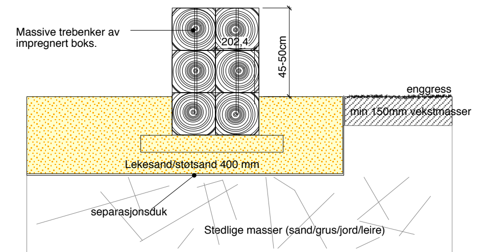
snitt 5 - sandleplass
