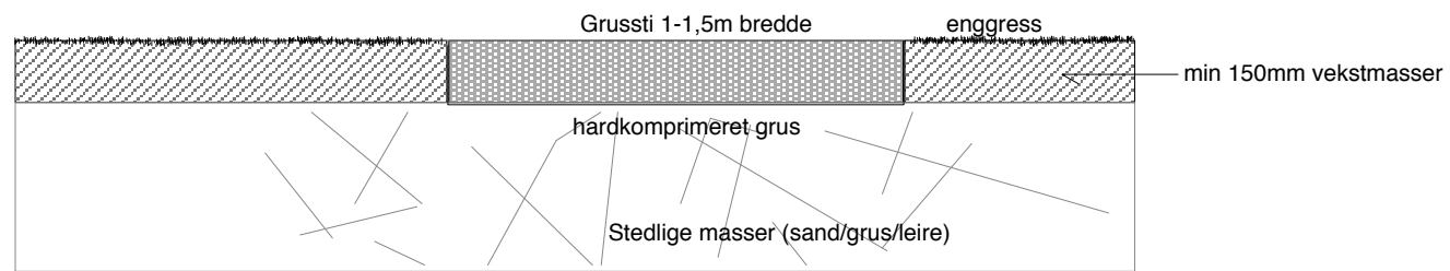
snitt 2 - gangsti
