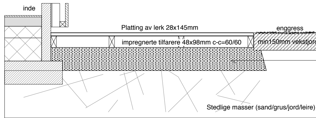
snitt 3 - treplattung
