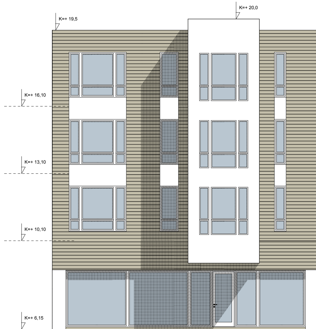
1:100 Fasade øst
