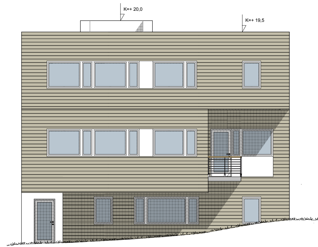
1:100 Fasade Vest
